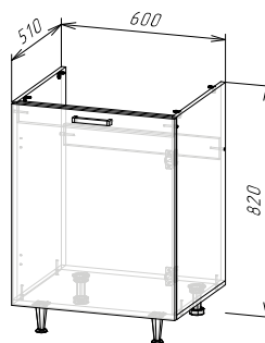
Корпус: ШНМ600/ШНМ1Д600 (490) (ШхВхГ) 600x820x510 мм Фасад: ЛДСП ФАСАД РИО NEW ШВ1Д600/ШН1Д600/ШНМ1Д600
