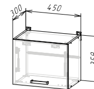
Корпус: ШВГ450/360 (ШхВхГ) 450х359х300 мм
