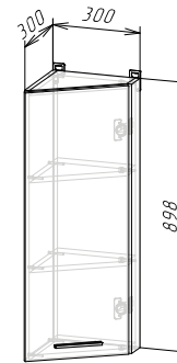
Корпус: ШВТД300/900 (ШхВхГ) 300х898х300 мм Фасад: ЛДСП ФАСАД РИО NEW ШВТД300/900
