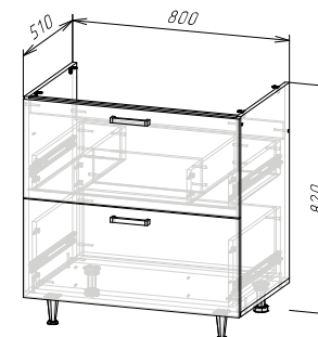
Корпус: ШНМ2ЯГ800(490) (ШхВхГ) 800х820х510 мм
