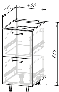
Корпус: ШН2ЯГ400(490) (ШхВхГ) 400х820х510 мм
