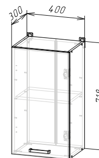
Корпус: ШВ400/ШВС400 (ШхВхГ) 400х718х300 мм
