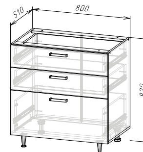
Корпус: ШНЗЯ800(490) (ШхВхГ) 800х820х510 мм
