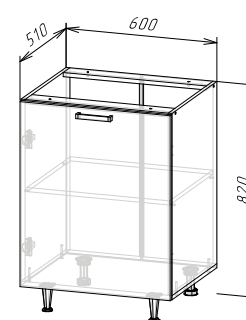
Корпус: ШН600/ШН1Д600 (490) (ШхВхГ) 600x820x510 мм Фасад: ЛДСП ФАСАД РИО NEW ШВ1Д600/ШН1Д600/ШНМ1Д600
