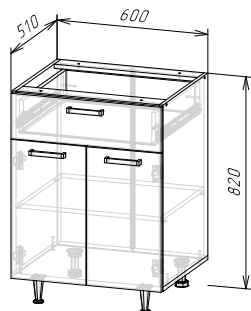
Корпус: ШН1Я600/ШН1Д1Я600(490) (ШхВхГ) 600х820х510 мм
