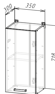
Корпус: ШВ350 (ШхВхГ) 350х718х300 мм
