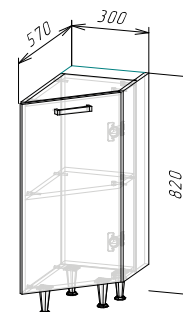
Корпус: ШНТД300 (ШхВхГ) 300х820х570 мм
