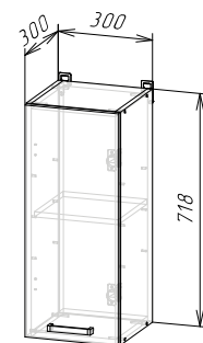
Корпус: ШВ300/ШВС300 (ШхВхГ) 300х718х300 мм
