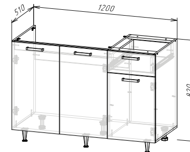
Корпус: ШН1Я1200(490) (ШхВхГ) 1200х820х510 мм
