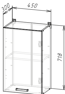
Корпус: ШВ450/ШВС450 (ШхВхГ) 450х718х300 мм
