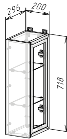
Корпус: ШВТД200 (ШхВхГ) 200х718х300 мм Фасад: ЛДСП ФАСАД РИО NEW ШВТД200/ШНТД200
