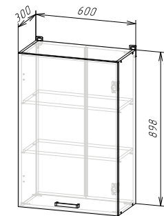
Корпус: ШВ600/900 / ШВС600/900 / ШВ1Д600/900 / ШВС1Д600/900 (ШхВхГ) 600х898х300 мм
