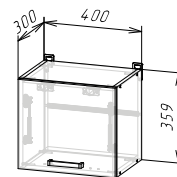
Корпус: ШВГ400/360 (ШхВхГ) 400х359х300 мм
