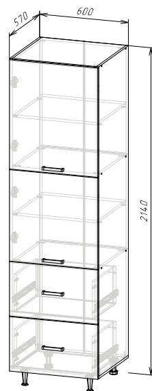
Корпус: ШП2Я600/ШП2Я600-1/ ШП2Я600-2 (ШхВхГ) 600х2140х570 мм Фасад: ЛДСП ФАСАД РИО NEW ШП2Я600-1
