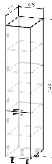
Корпус: ШП400/ШП400-1 (ШхВхГ) 400x2140x570 мм Фасад: ЛДСП ФАСАД РИО NEW ШП400-1
