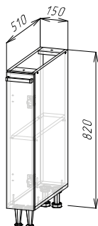
Корпус: ШН150(490) (ШхВхГ) 150x820x510 мм Фасад: ЛДСП ФАСАД РИО NEW ШВ150/ШН150
