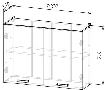
Корпус: ШВ1000/ШВС1000 (ШхВхГ) 1000х718х300 мм
