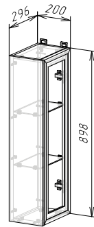
Корпус: ШВТД200/900 (ШхВхГ) 200х898х300 мм Фасад: ЛДСП ФАСАД РИО NEW ШВТД200/900
