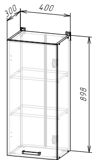
Корпус: ШВ400/900 / ШВС400/900 (ШхВхГ) 400х898х300 мм
