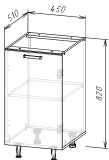
Корпус: ШН450(490) (ШхВхГ) 450x820x510 мм Фасад: ЛДСП ФАСАД РИО NEW ШВ450/ШН450
