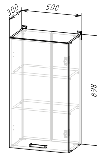
Корпус: ШВ500/900 / ШВС500/900 (ШхВхГ) 500х898х300 мм
