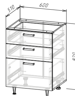
Корпус: ШНЗЯ600(490) (ШхВхГ) 600х820х510 мм
