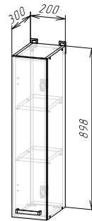
Корпус: ШВ200/900 (ШхВхГ) 200х898х300 мм
