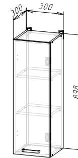
Корпус: ШВ300/900 / ШВС300/900 (ШхВхГ) 300х898х300 мм
