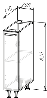
Корпус: ШН200(490) (ШхВхГ) 200x820x510 мм Фасад: ЛДСП ФАСАД РИО NEW ШВ200/ШН200
