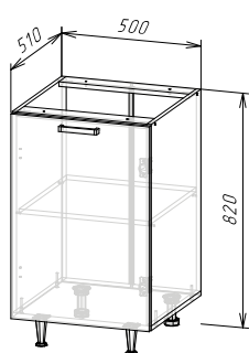
Корпус: ШН500(490) (ШхВхГ) 500x820x510 мм Фасад: ЛДСП ФАСАД РИО NEW ШВ500/ШН500/ШНМ500
