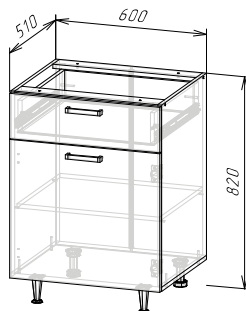
Корпус: ШН1Я600/ШН1Д1Я600(490) (ШхВхГ) 600х820х510 мм
