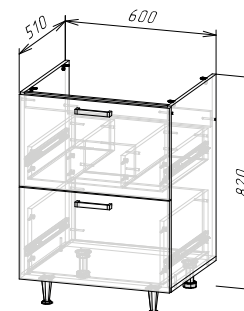
Корпус: ШНМ2ЯГ600(490) (ШхВхГ) 600х820х510 мм
