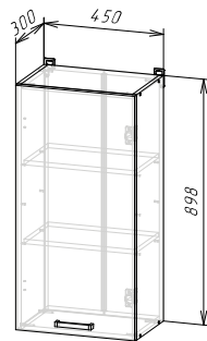
Корпус: ШВ450/ШВС450 (ШхВхГ) 450х898х300 мм
