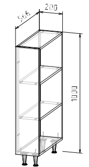
Корпус: ТР 1000 (ШхВхГ) 200х1000х566 мм
