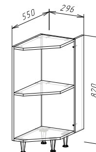
Корпус: ШНТ300 (ШхВхГ) 296х820х550 мм
