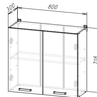
Корпус: ШВ800/ШВС800 (ШхВхГ) 800х718х300 мм
