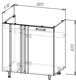
Корпус: ШНУ1000(490) (ШхВхГ) 800х820х510 мм
