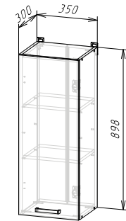
Корпус: ШВ350/900 (ШхВхГ) 350х898х300 мм
