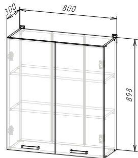
Корпус: ШВ800/900/ШВС800/900 (ШхВхГ) 800х898х300 мм
