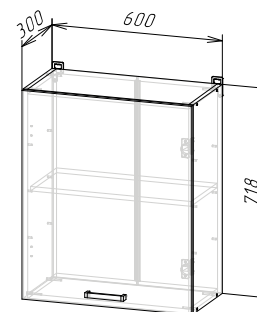
Корпус: ШВ600/ШВС600/ ШВ1Д600/ШВС1Д600 (ШхВхГ) 600х718х300 мм
