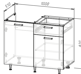
Корпус: ШН1Я1000(490) (ШхВхГ) 1000х820х510 мм
