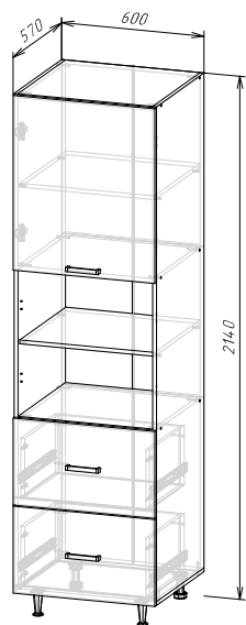
Корпус: ШП2Я600/ШП2Я600-1/ ШП2Я600-2 (ШхВхГ) 600х2140х570 мм Фасад: ЛДСП ФАСАД РИО NEW ШП2Я600
