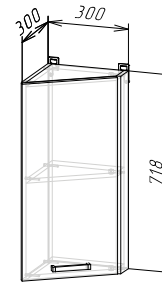
Корпус: ШВТД300 (ШхВхГ) 300х718х300 мм Фасад: ЛДСП ФАСАД РИО NEW ШВТД300
