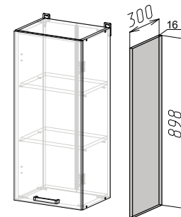
ЛДСП ФАСАД РИО NEW БФП (898х300) (ШхВхГ) 898х300х16 мм
