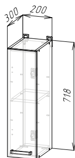
Корпус: ШВ200 (ШхВхГ) 200х718х300 мм
