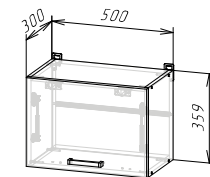
Корпус: ШВГ500/360 / ШВГС500/360 (ШхВхГ) 500х359х300 мм
