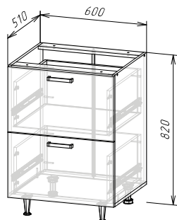
Корпус: ШН2ЯГ600(490) (ШхВхГ) 600х820х510 мм
