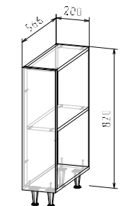
Корпус: ТР 820 (ШхВхГ) 200х820х566 мм
