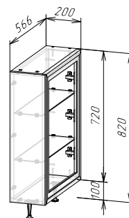
Корпус: ШНТД200 (ШхВхГ) 200х820х566 мм
