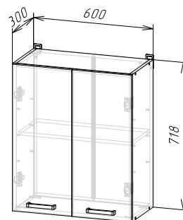
Корпус: ШВ600/ШВС600/ ШВ1Д600/ШВС1Д600 (ШхВхГ) 600х718х300 мм
