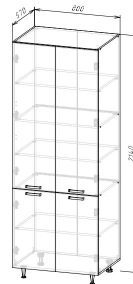
Корпус: ШП800/ШП800 (ШхВхГ) 800х2140х570 мм Фасад: ЛДСП ФАСАД РИО NEW ШП800
