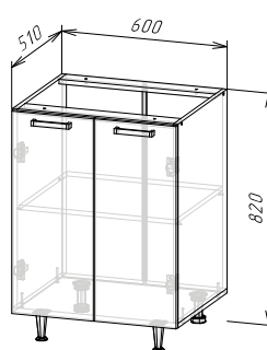
Корпус: ШН600/ШН1Д600 (490) (ШхВхГ) 600x820x510 мм Фасад: ЛДСП ФАСАД РИО NEW ШВ600/ШН600/ШНМ600
