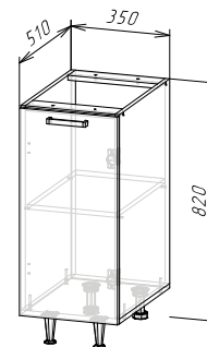
Корпус: ШН350(490) (ШхВхГ) 350x820x510 мм Фасад: ЛДСП ФАСАД РИО NEW ШВ350/ШН350
