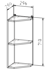
Корпус: ШВТ 300 (ШхВхГ) 296х718х280 мм
