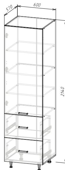
Корпус: ШП2Я600/ШП2Я600-1/ ШП2Я600-2 (ШхВхГ) 600х2140х570 мм Фасад: ЛДСП ФАСАД РИО NEW ШП2Я600-2
