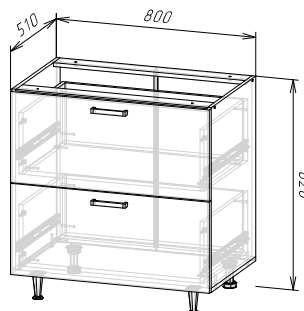
Корпус: ШН2ЯГ800(490) (ШхВхГ) 800х820х510 мм
