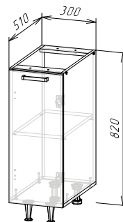
Корпус: ШН300(490) (ШхВхГ) 300x820x510 мм Фасад: ЛДСП ФАСАД РИО NEW ШВ300/ШН300
