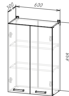
Корпус: ШВ600/900 / ШВС600/900 / ШВ1Д600/900 / ШВС1Д600/900 (ШхВхГ) 600х898х300 мм
