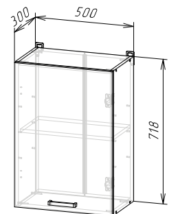
Корпус: ШВ500/ШВС500 (ШхВхГ) 500х718х300 мм
