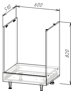
Корпус: ШНВТ600(490) (ШхВхГ) 600х820х510 мм
