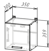
Корпус: ШВГ350/360 (ШхВхГ) 350х359х300 мм
