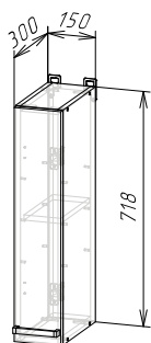
Корпус: ШВ150 (ШхВхГ) 150х718х300 мм
