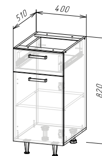
Корпус: ШН1Я400(490) (ШхВхГ) 400x820x510 мм Фасад: ЛДСП ФАСАД РИО NEW ШН1Я400
