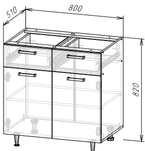
Корпус: ШН2Я800(490) (ШхВхГ) 800х820х510 мм
