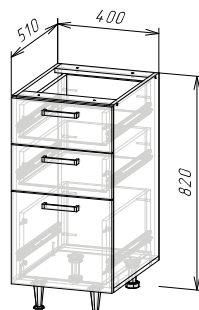
Корпус: ШНЗЯ400(490) (ШхВхГ) 400х820х510 мм
