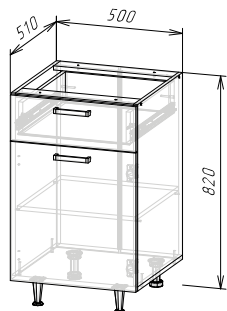
Корпус: ШН1Я500(490) (ШхВхГ) 500х820х510 мм
