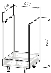
Корпус: ШНВТ450(490) (ШхВхГ) 450х820х510 мм
